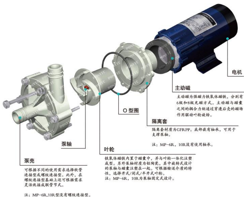
结构图
